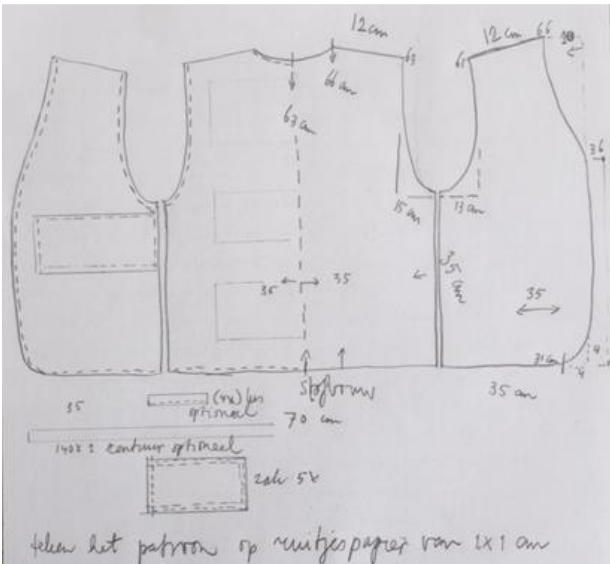
Afbeelding 1: Het patroon met alle afmetingen. Let op: check voor de zakken de maat van de coldpacks die je hebt gekocht.
